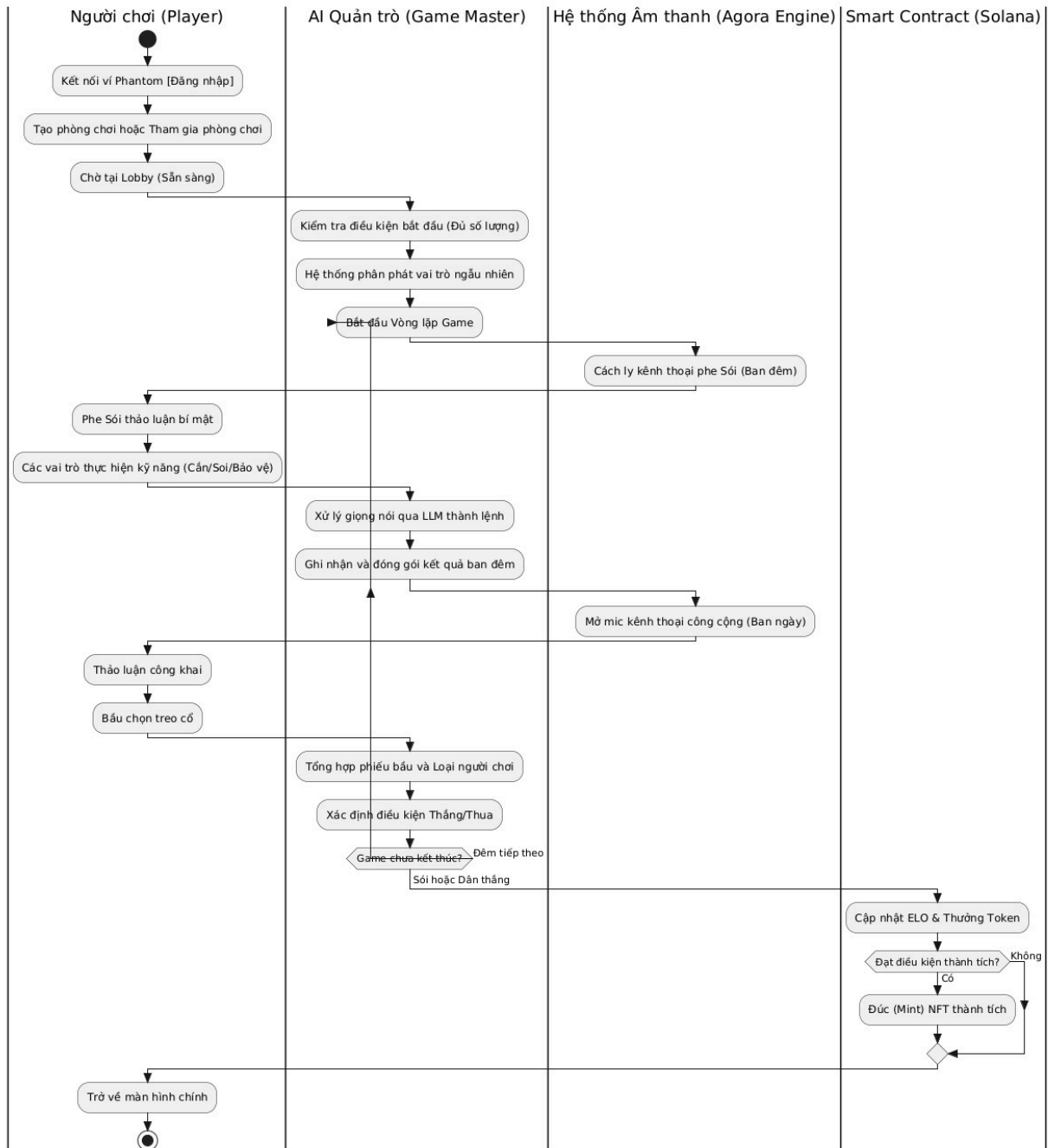
Sơ đồ Hoạt động (Activity Diagram) - Hệ thống Game Ma Sói
